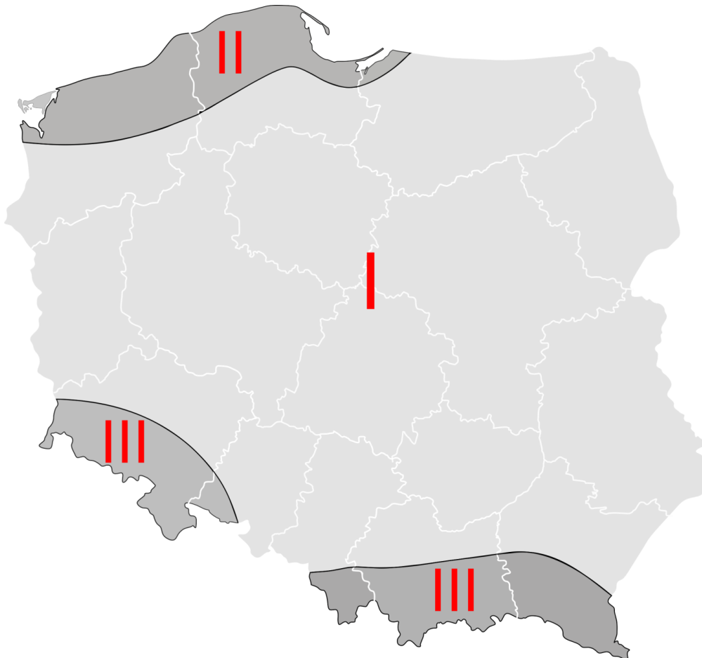
mapa stref obciążenia wiatrem wg PN-EN 1991-1-4:2008
